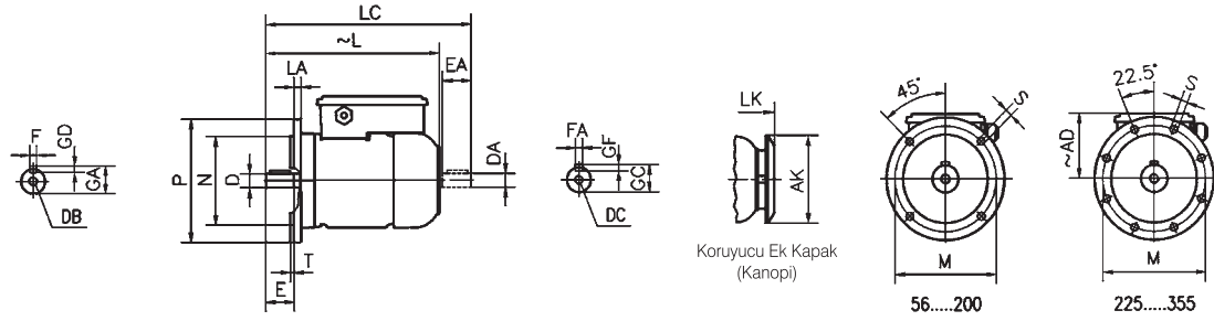
FLANŞLI MOTOR (BİÇİM "A" - DIN EN 50 347) - B5, V1, V3
